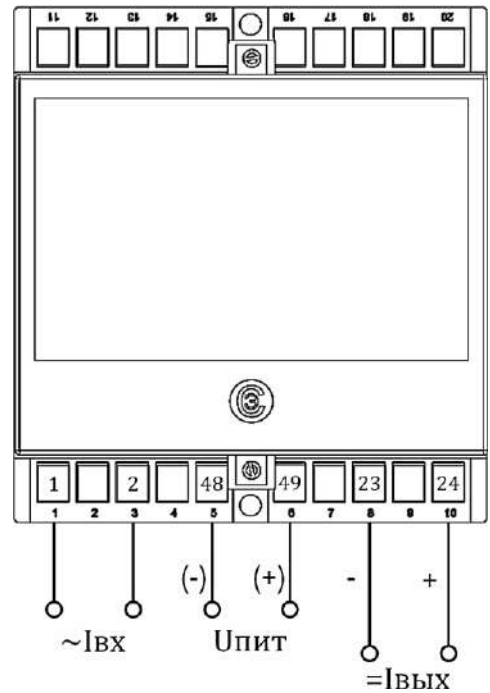
Копус Е20 (1 вход, 1 аналоговый выход)
