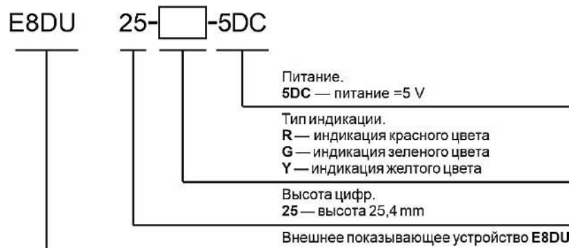
Рисунок 2 – Схема условного обозначения E8DU (поставляется в комплекте для ИП с портом для внешнего показывающего устройства)
