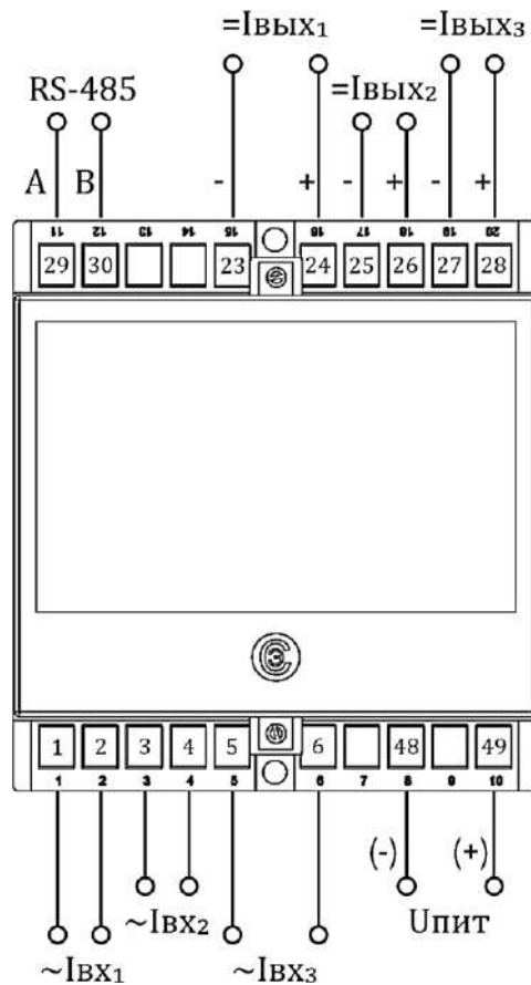
Копус E20 (3 входа, 3 аналоговых выхода, 1 порт RS-485)
