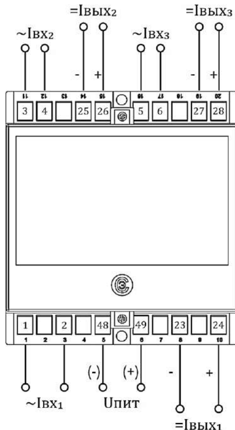
Корпус E20 (3 входа, 3 аналоговых выхода)
