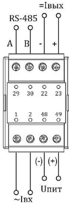
Копус М8 (1 вход, 1 аналоговый выход, 1 порт RS-485)
