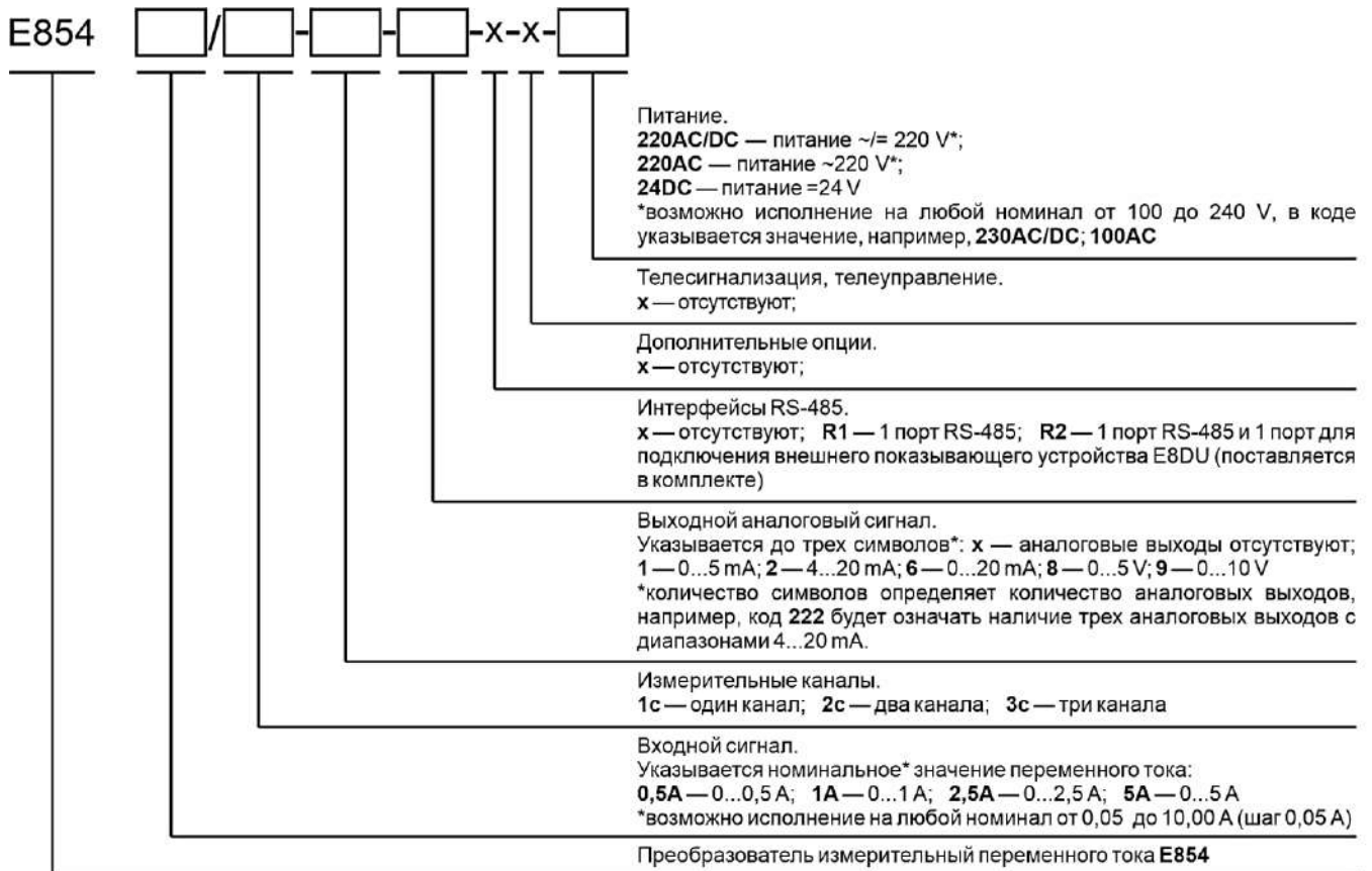
Рисунок 1 – Схема условного обозначения ИП (подробное описание корпусов и возможных исполнений указано в п. 2.16)
