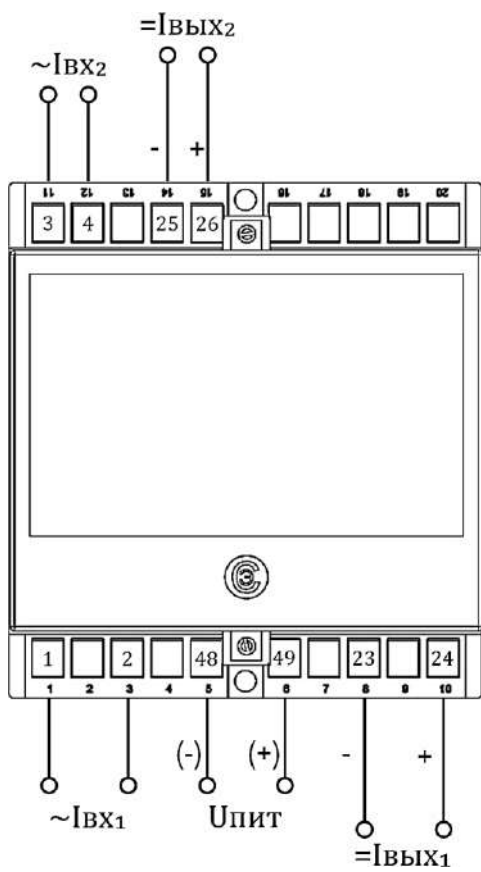
Корпус E20 (2 входа, 2 аналоговых выхода)
