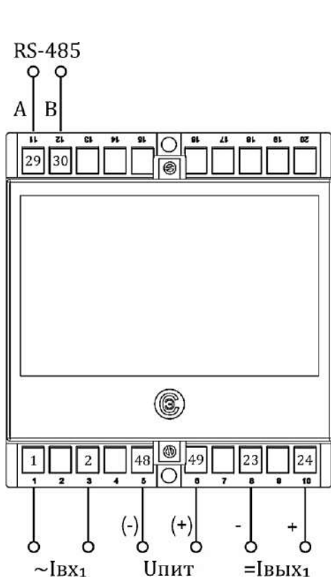
Копуса E20 (1 вход, 1 аналоговый выход, 1 порт RS-485)
