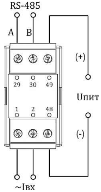
Копус М6 (1 вход, 1 порт RS-485)
