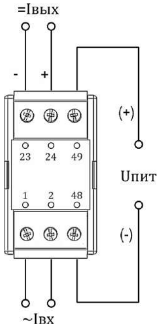
Копус М6 (1 вход, 1 аналоговый выход)
